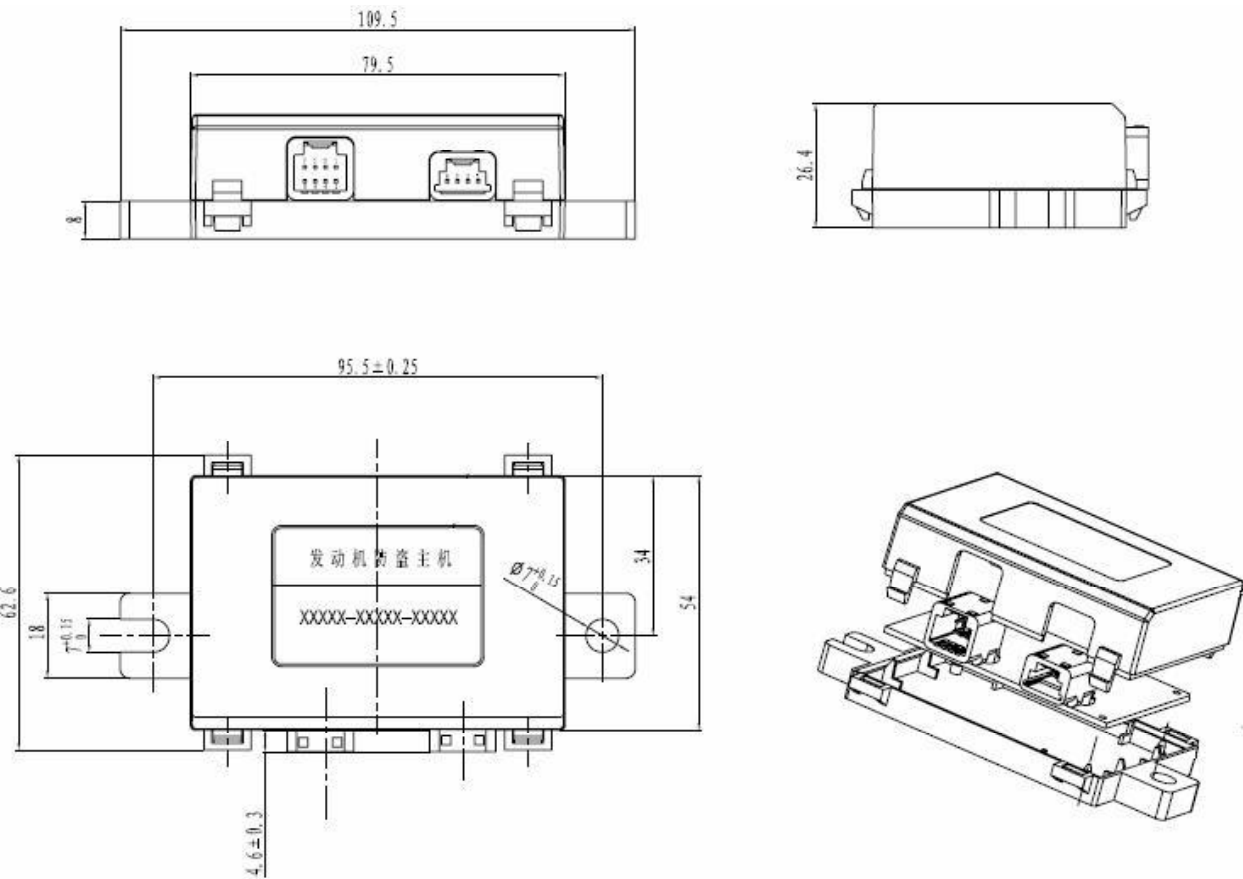
图1 外壳尺寸图
